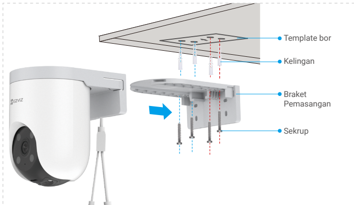
Gbr. 1 Pemasangan pada Plafon
